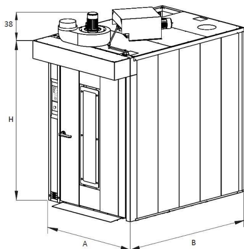
ROTOR VORTEX - LFRNP | LFRNPE
